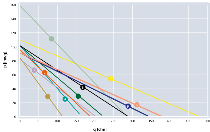
cfm vs inwg
